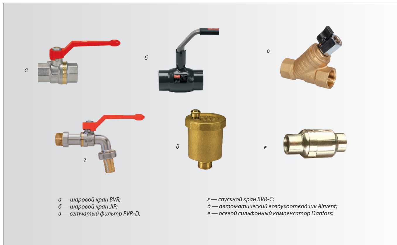
Рис. 22. Трубопроводная арматура.
