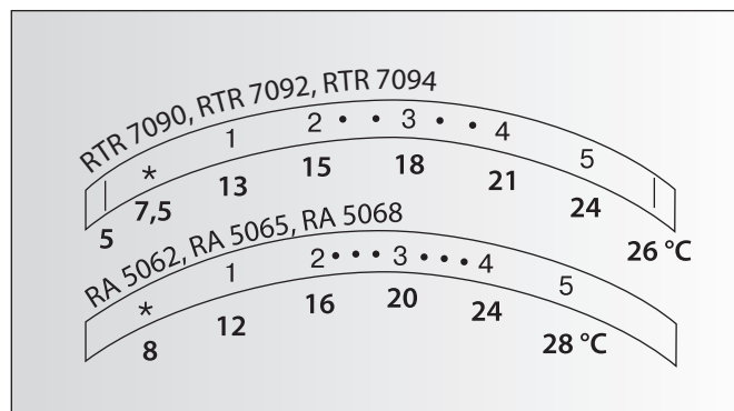
Рис. 4. Шкалы температурной настройки термоэлементов типа RTR.
