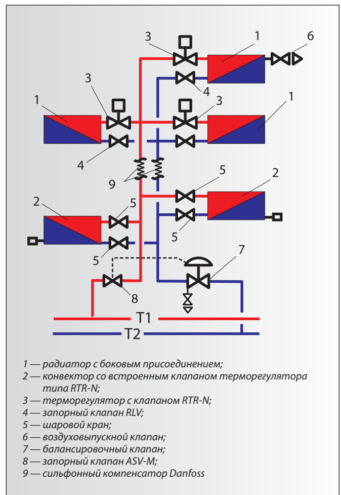
Рис. 31. Стояк двухтрубной автоматизированной системы отопления с нижним расположением магистралей.
