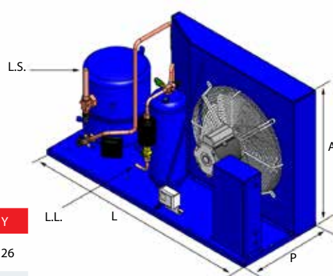
Vista isométrica
