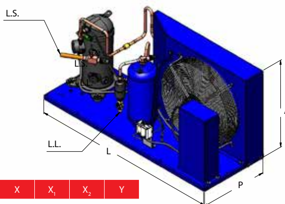
Vista isométrica
