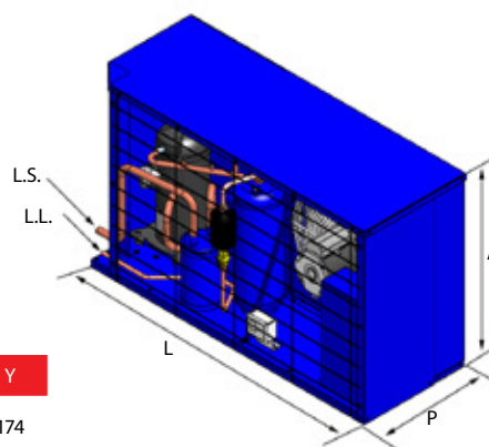
Vista isométrica
