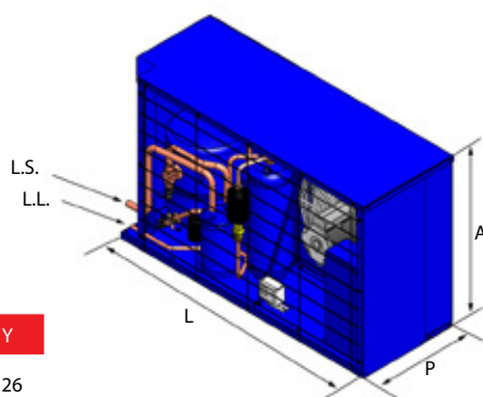
Vista isométrica
