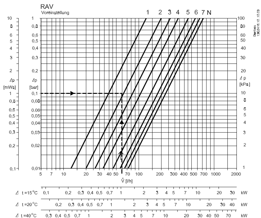
RAV 10-15-20 Auslegungsdigramm.
