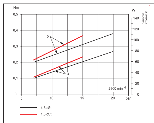
工作扭矩
