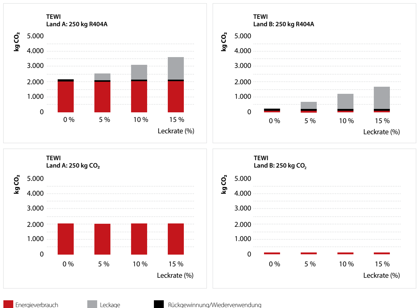
Abbildung 19: Verhältnis zwischen direkten und indirekten Auswirkungen der Kälteanlage
