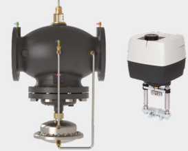
PICV-1: AB-QM + AME 655
