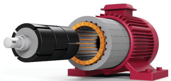
PM-Motor mit oberflächenmontierten Magneten
