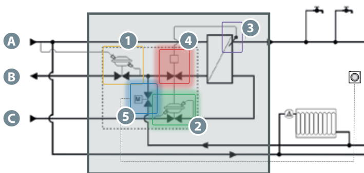
(A) Stadswarmte retour (B) Stadswarmte aanvoer (C) Koud drinkwater
