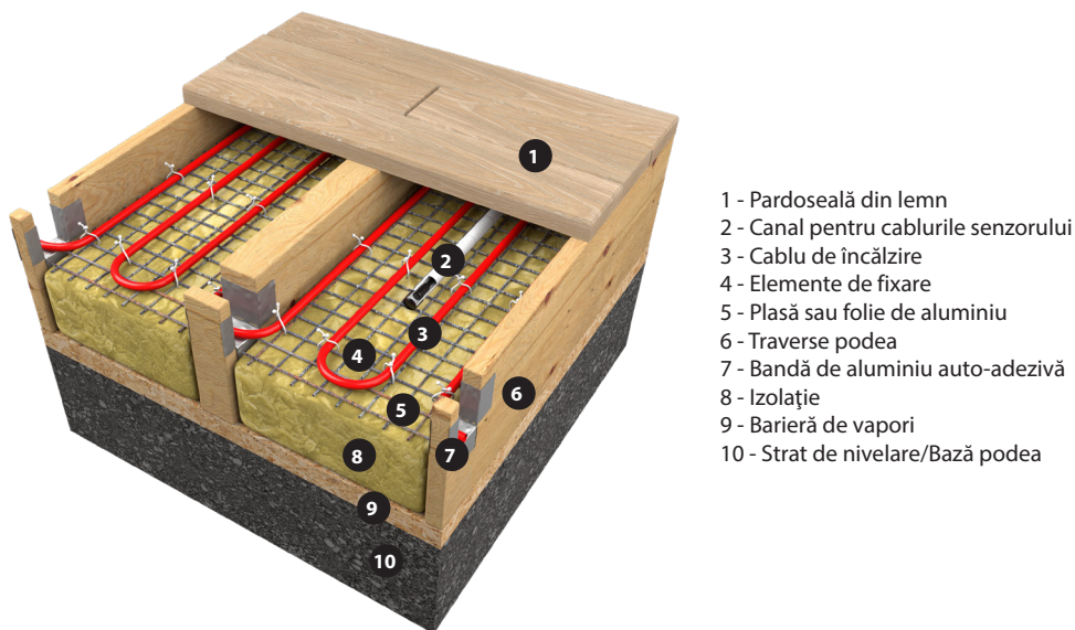
Fig. 13. Podea din lemn pe traverse
