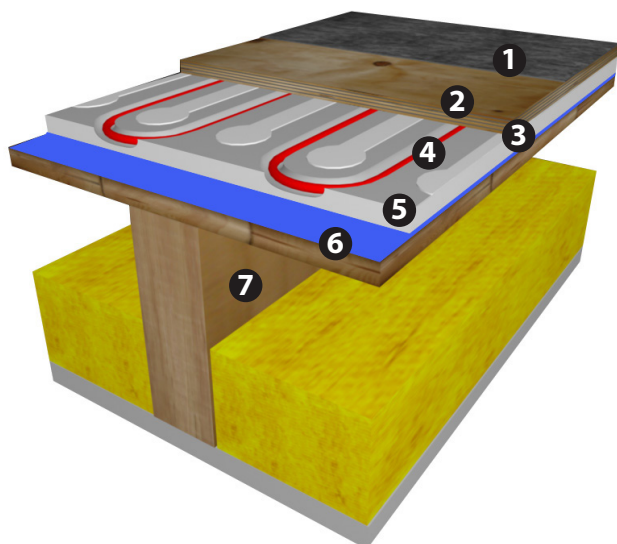
Fig. 22. Încălzire în pardoseală cu panourile DEVicell™ în podele existente din lemn
