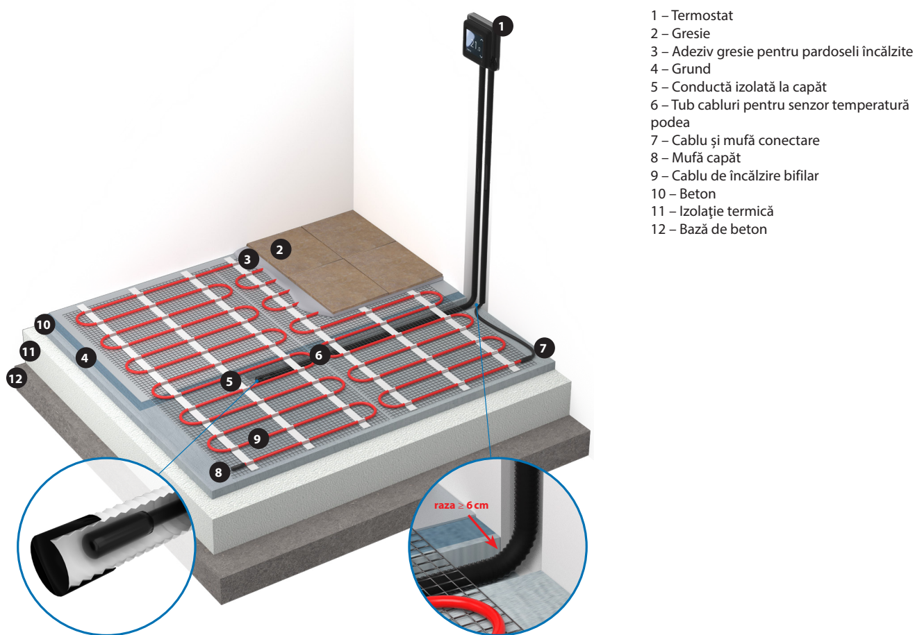
Fig. 6. Construcție pardoseală subțire cu covoraș de încălzire subțire cu cabluri conductoare bifilare
