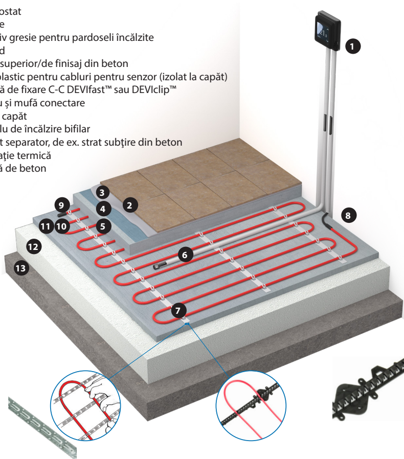
Fig. 4. Încălzire prin cabluri în podea de beton cu cablu fixat cu bandă de fixare C-C DEVIfast™ sau DEVclip™.
