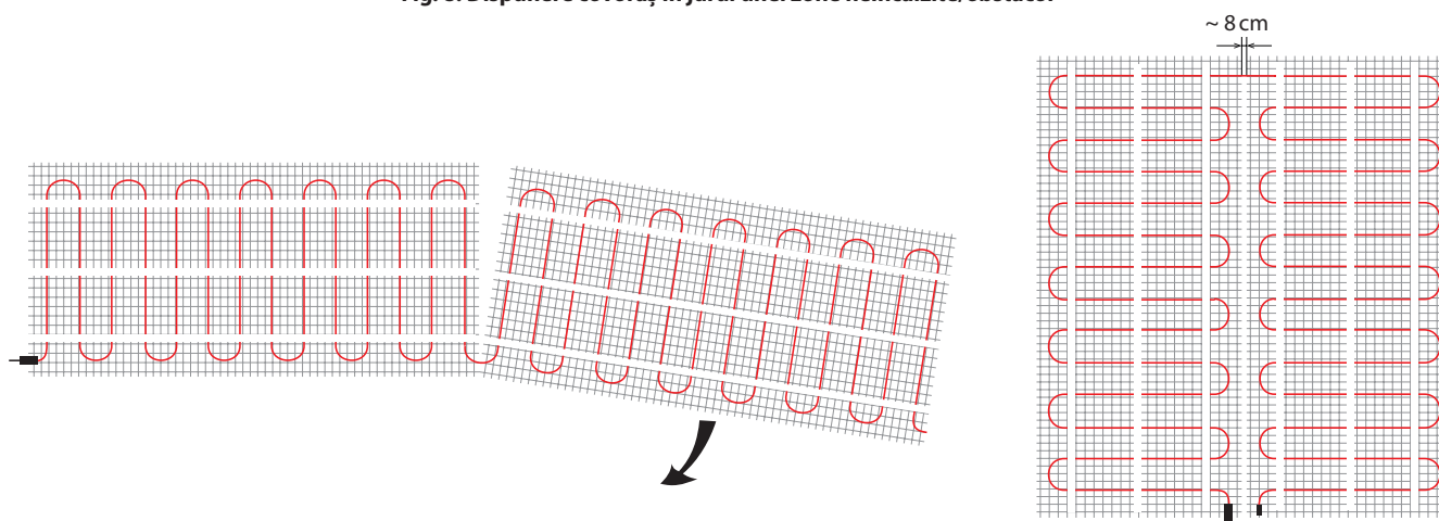
Fig. 9. Covorașele de încălzire pot fi foarte ușor adaptate la forma suprafeței de încălzit. Exemplu de mai sus: plasarea DEVImat™ 150T 50 x 300 cm pe 100 x 150 cm.
