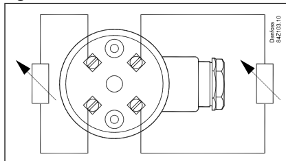
Figura 2: Conexión eléctrica
