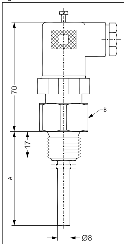
Figura 3: Dimensiones
