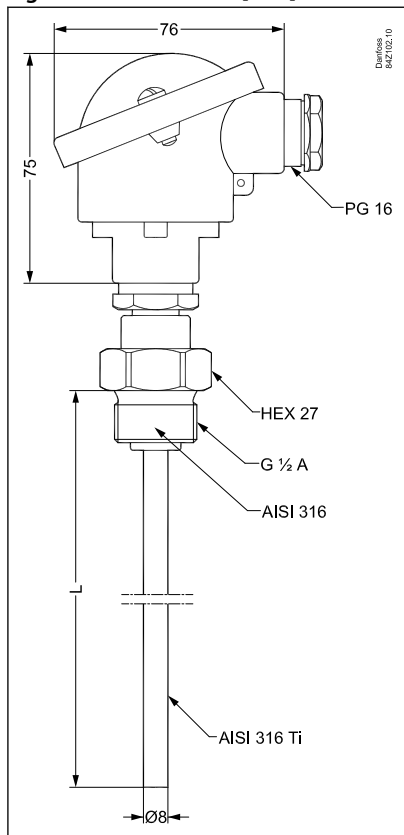
Figura 1: Dimensiones [mm]
