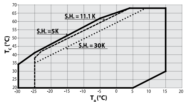
R410A - SH
