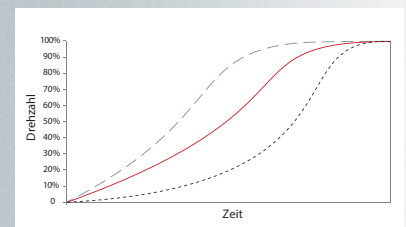
Drei Startprofile für die Adaptive Beschleunigungsregelung (AAC); frühe, konstante und späte Beschleunigung
