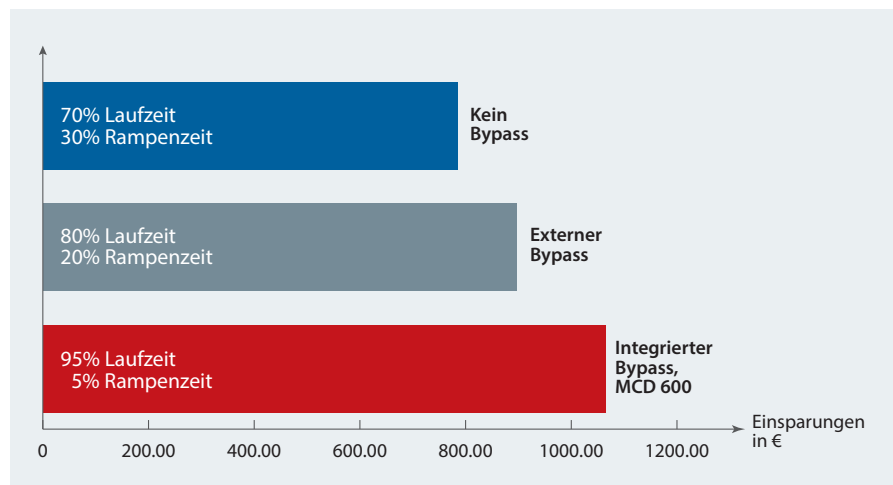
Kostenersparnis durch Bypass, was den vorteilhaften Einspareffekt von erhöhter Laufzeit und verkürzter Rampenzeit zeigt.
