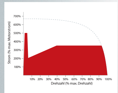
Konstantstrom-/Stromrampe – hier mit Kickstart dargestellt
