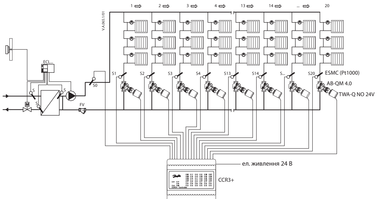
Рис. 2. Обмеження максимальної витрати з регулюванням температури теплоносія на виході стояків у однотрубній системі зі змінним гідравлічним режимом (термогідравлічне балансування)
