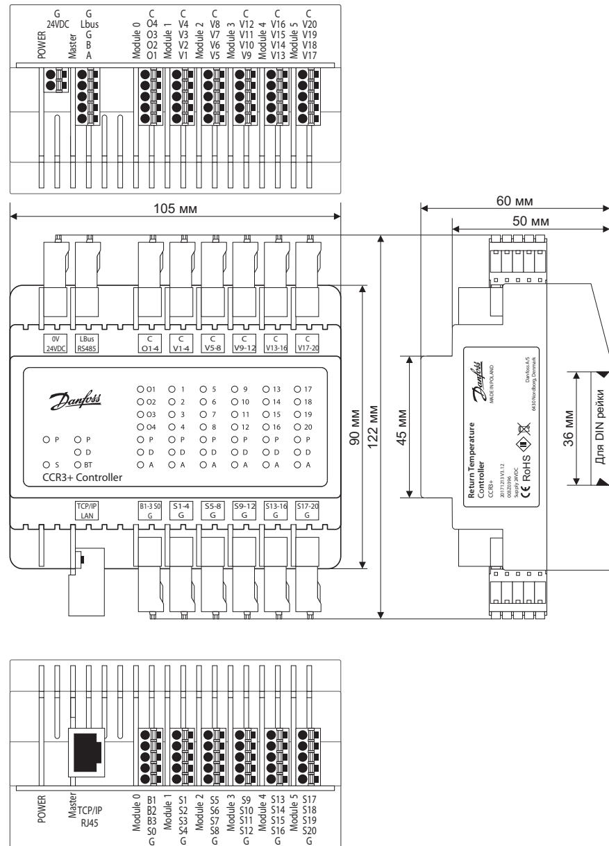
Рис. 3. Схема підключення контролера CCR3+
