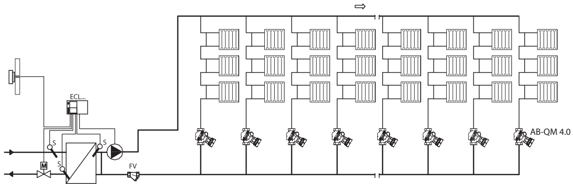
Рис. 1. Стабілізація витрати в однотрубній системі опалення з постійним гідравлічним режимом
