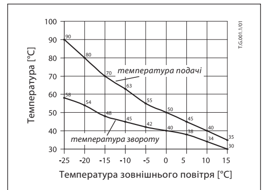
Рис. 2. Графік залежності температур подаючого та зворотного теплоносія від температури зовнішнього повітря
