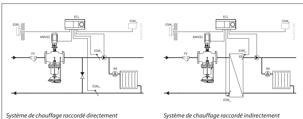
Système de chauffage raccordé directement
