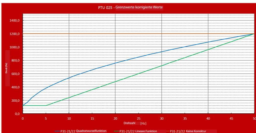
Druck-/Drehzahlkurveneinstellungen
