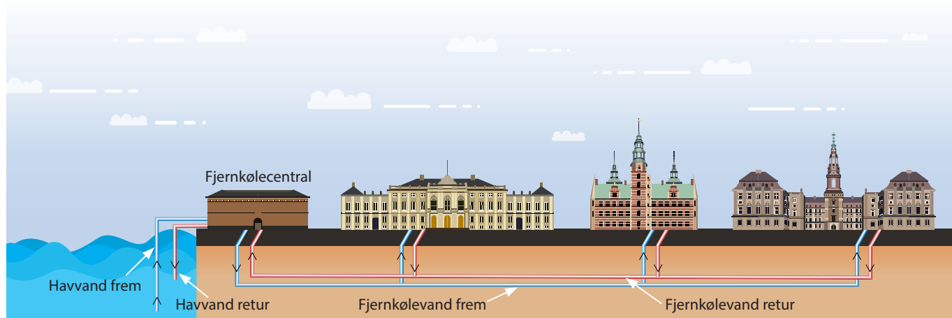
Principskitse af fjernkølesystemet hos HOFOR
