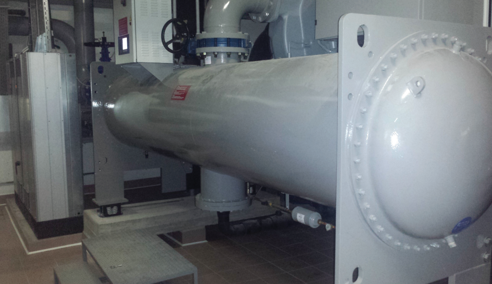
Twee 19 XR compressoren met een koelvermogen van 2245 kW en een elektrisch vermogen van 375 kW ondersteunen nu het koelsysteem.
