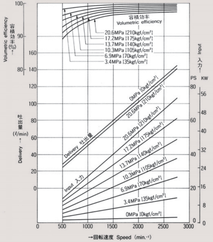
PC6 押しのけ容積 52.9cm 3 /rev. Displacement
