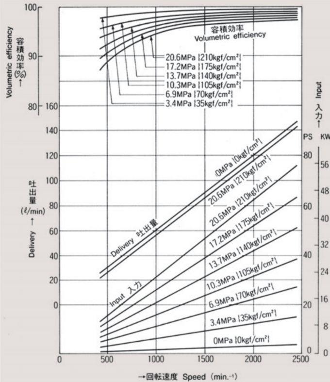
PC7 押しのけ容積 60.1cm 3 /rev. Displacement
