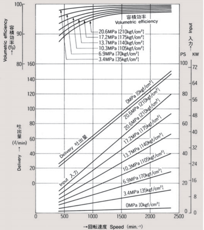
PC8 押しのけ容積 63.6cm 3 /rev. Displacement
