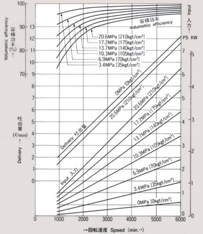
PA2 押しのけ容積 2.07cm 3 /rev. Displacement
