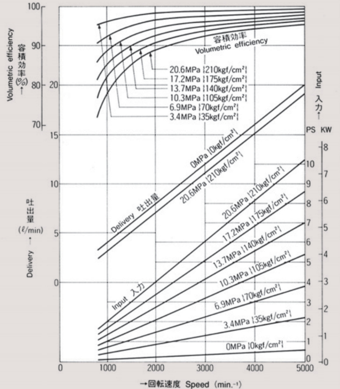
PA4 押しのけ容積 4.06cm 3 /rev. Displacement
