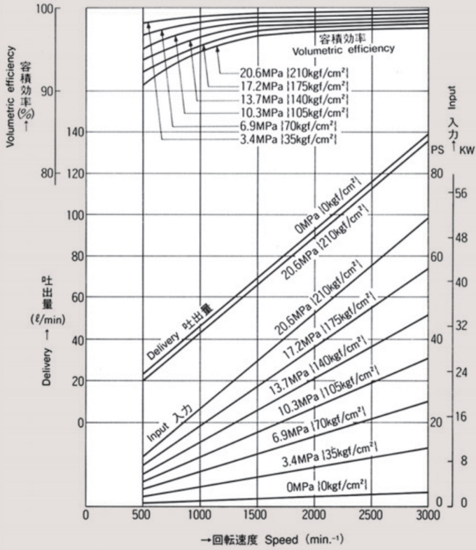
PC5 押しのけ容積 45.9cm 3 /rev. Displacement
