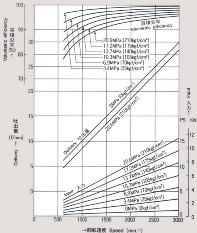
PB2 押し のけ容積 10.0cm 3 /rev. Displacement
