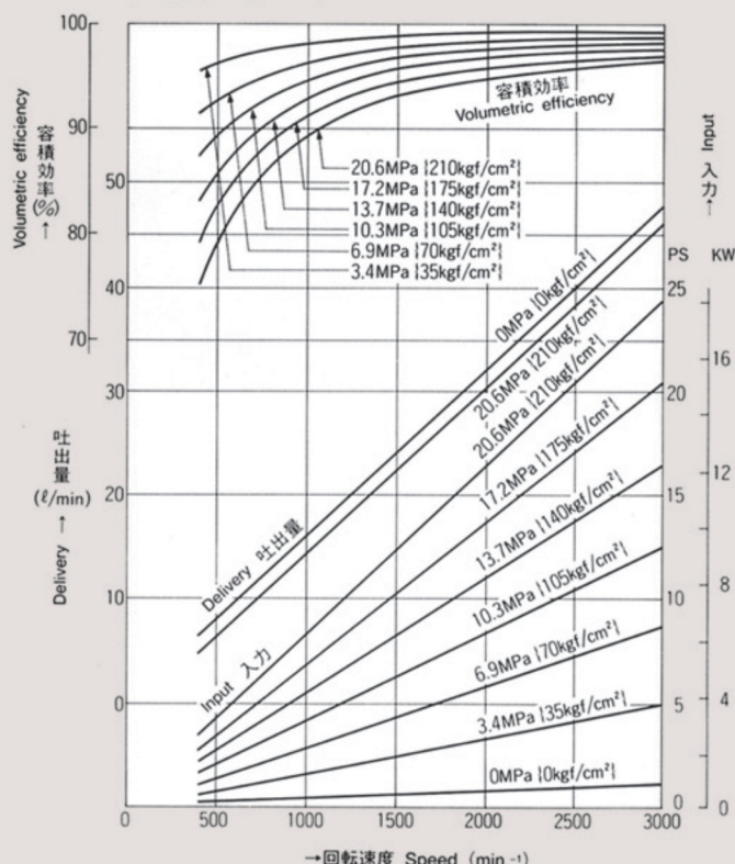
PB4 押し のけ容積 16.0cm 3 /rev. Displacement
