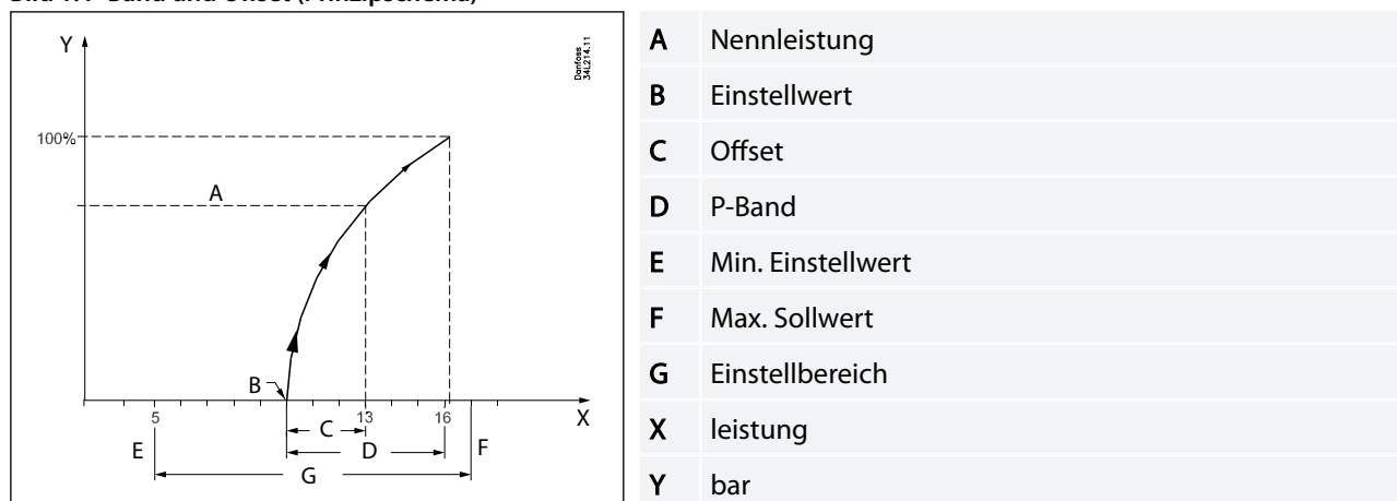
Bild 1: P-Band und Offset (Prinzipschema)
