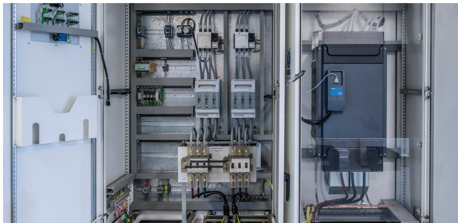
De configuratie van de schakelkasten na de vervanging met rechts de VACON® frequentieomvormer. De nieuwe omvormer neemt veel minder ruimte in dan zijn voorganger.
