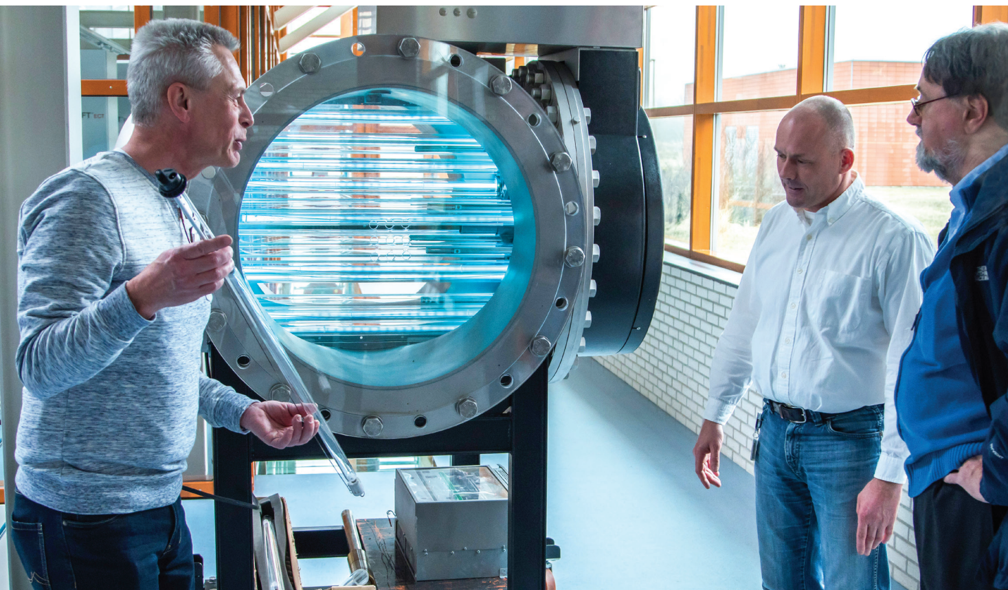
Bedrijfsvoerder Rob van der Hulst (links) beschrijft de functie, werking en configuratie van de UV-lampen. UV-licht breekt micro-organismen en resten van pesticiden en medicijnen af.
