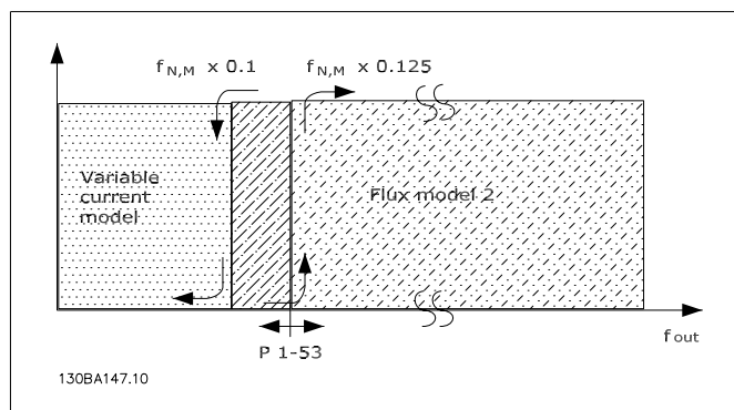
Obrázek 2.3: Par. 1-00 = [0] Otáčková zp. vazba Par. 1-01 = [2] Vektorové, bezsním.
