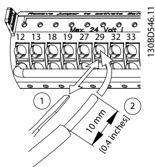
Illustration 5.38 Tilslutning af bløde styreledninger
