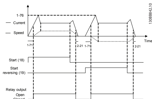
Illustration 8.5 Mekanisk bremsestyring
