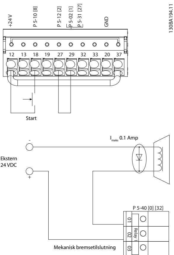
Illustration 8.8 Ledningskonfiguration for moment- og stopgrænse
