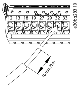
Illustration 5.37 Tilslutning af faste styreledninger
