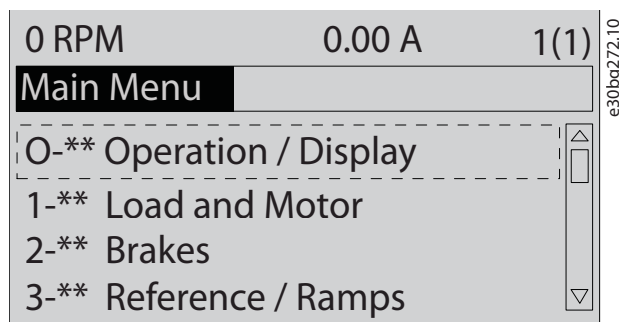
Illustration 3.7 Hovedmenu-skærbillede
