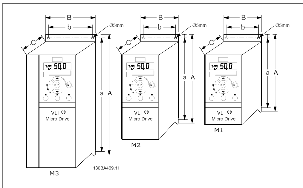
Obrázek 2.3: Mechanické rozměry.
