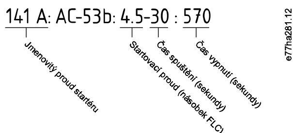
Obrázek 2: Formát AC53b
