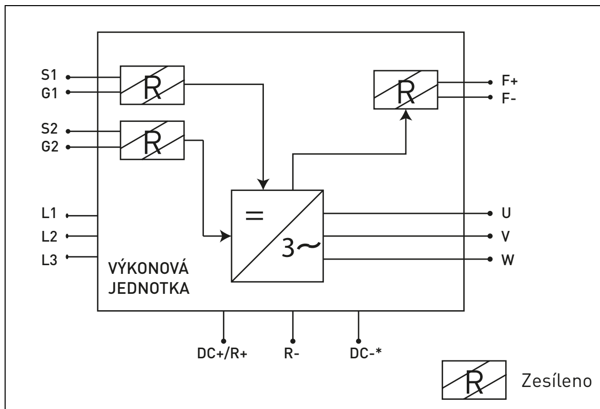
Obrázek 71. Princip funkce STO. (*) Pouze pro MU3.
