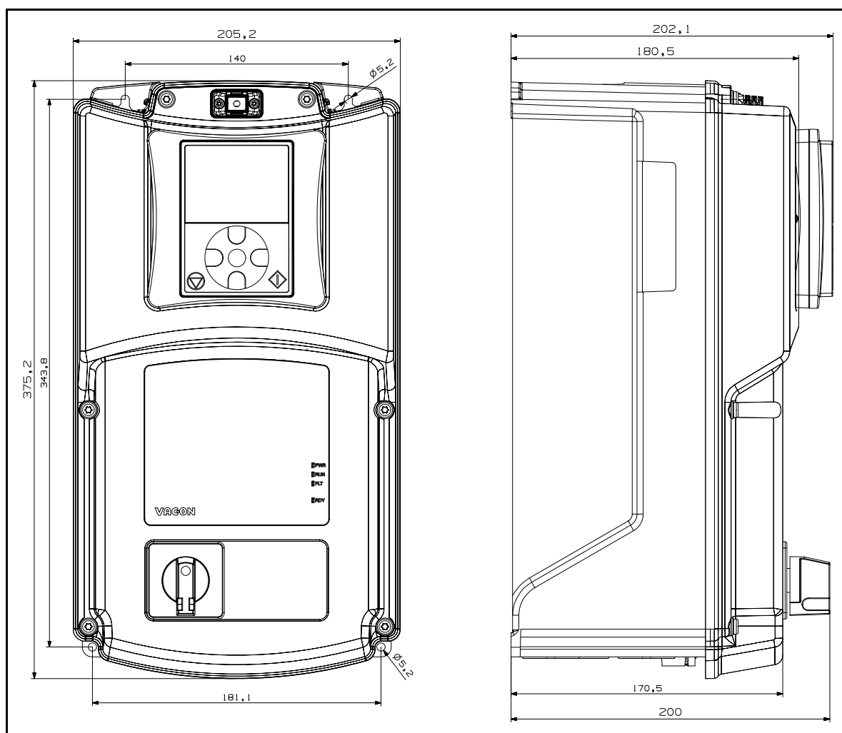
Obrázek 10. VACON® 20 X, MU3.
