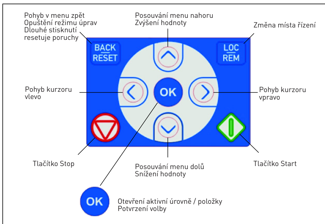
Obrázek 50. Tlačítka panelu.
