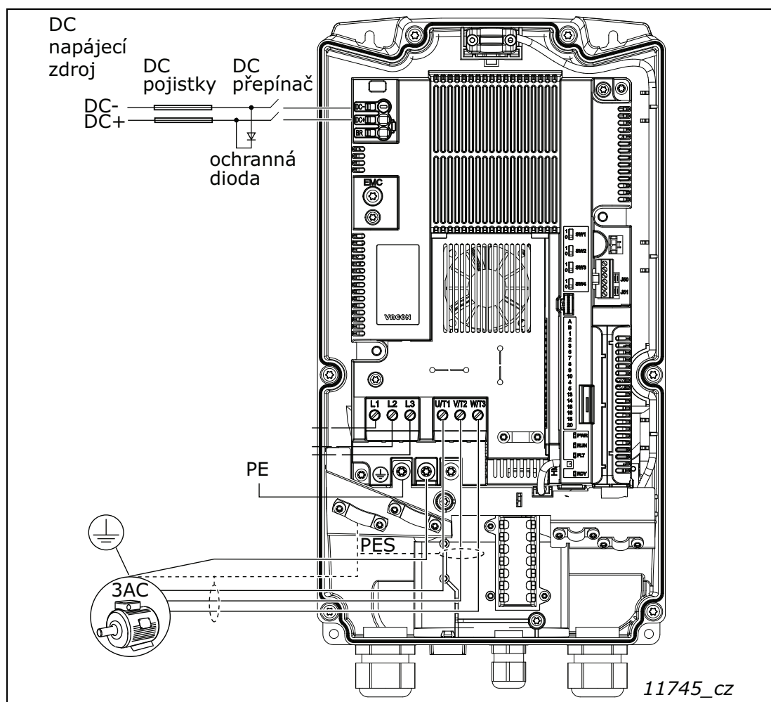
Obrázek 78. Příklad připojení napájení: MU3.
