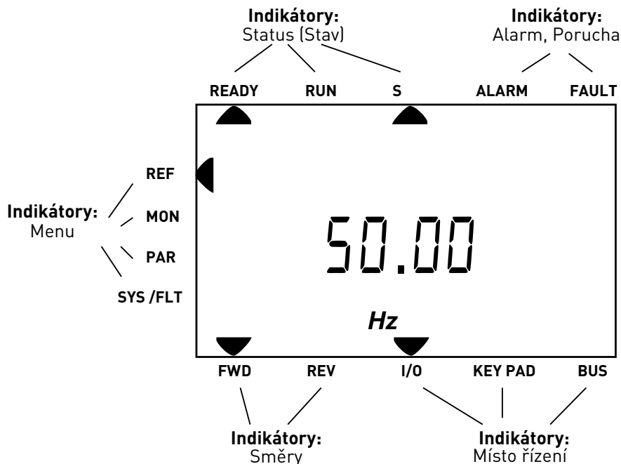
Obrázek 51. Displej panelu.
