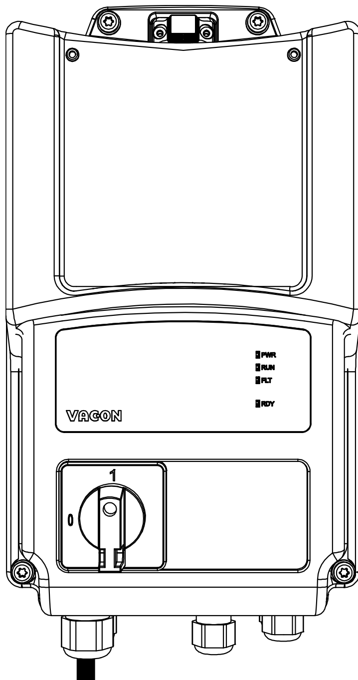
Obrázek 66. Namontujte plastový kryt.
