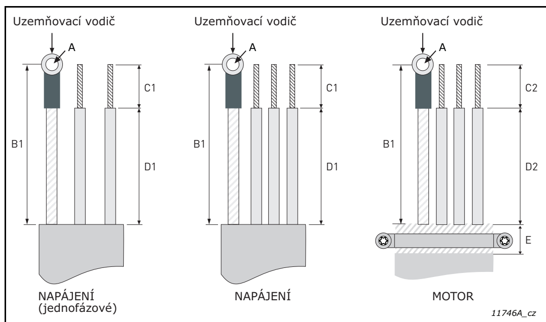
Obrázek 19. Odizolování kabelů.
