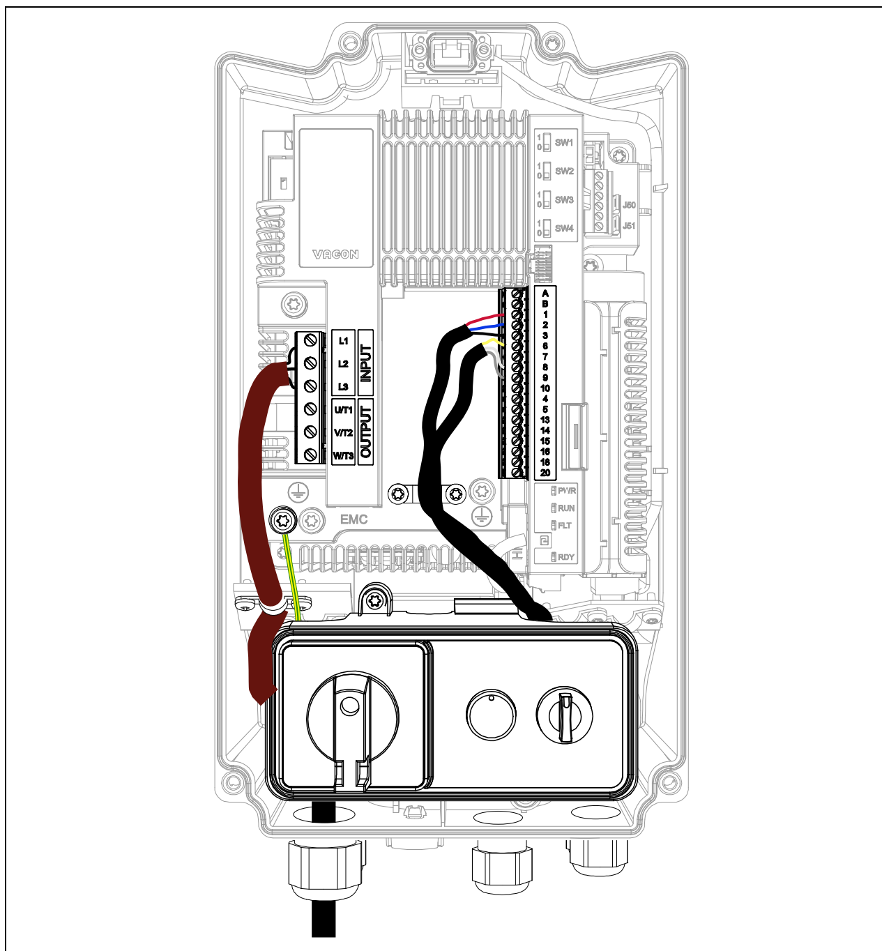
Obrázek 69. Připojený jednoduchý ovládací panel (příklad s třífázovým MU2).
