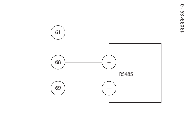
Illustration 5.39 Schéma de câblage de la communication série
