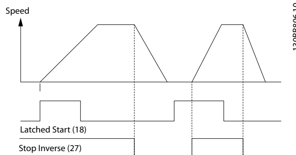
Illustration 8.2 Démarrage par impulsion/arrêt
