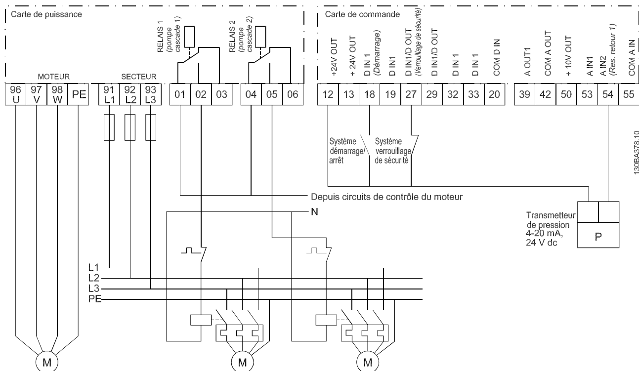
Illustration 8.6 Schéma de câblage du contrôleur de cascade
