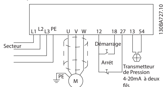
Illustration 8.4 Câblage de l'application de pompe submersible
