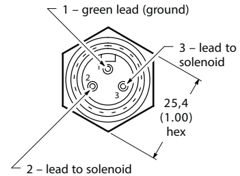
KTG4V-3S-**-M-FPA3
