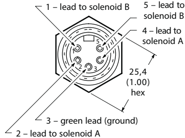
KDG4V-3S-*C-M-FPA5
