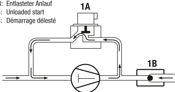
Bild 4: Normalbetrieb (Vollast) Fig. 4: Normal operation (full load) Fig. 4: Fonctionnement normal (à pleine charge)
