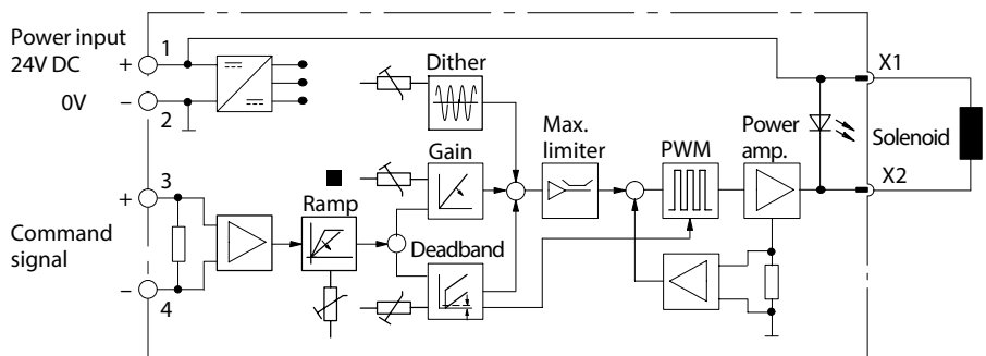
EHH-AMP-702-D/J/K-2*
