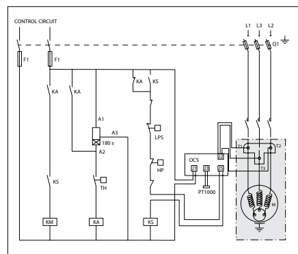
Krettschema utan nedsugningscykel
