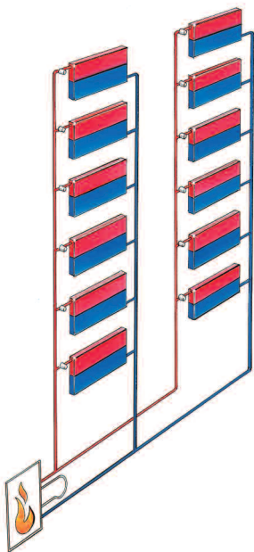
Korrekte Wasserverteilung durch voreinstellbare Ventile
