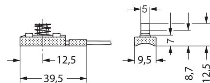
Sonde de température d'applique
