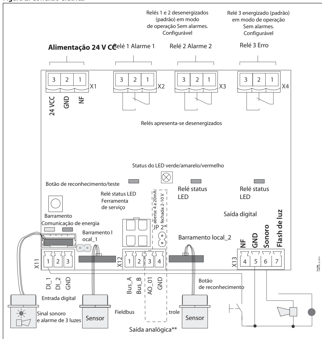
Figura 2: Conexão elétrica
