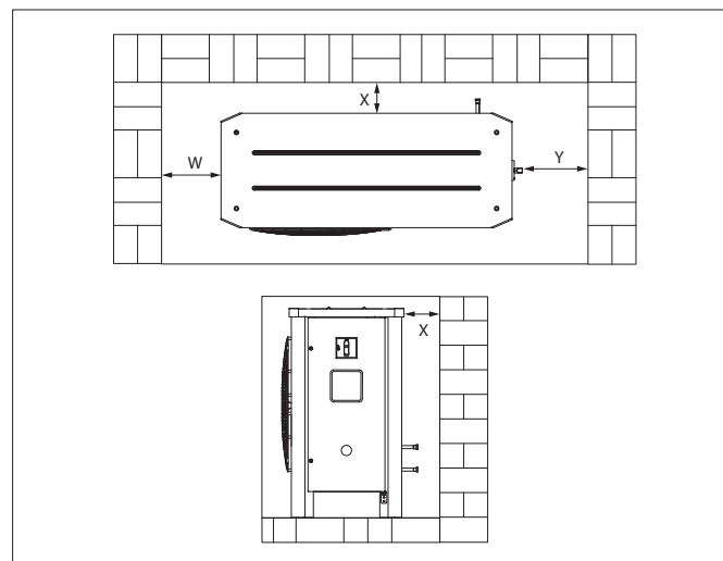
Abbildung 1: Mindestmontageabstände
