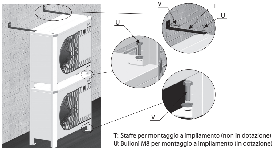
Figura 2: Montaggio a impilamento
