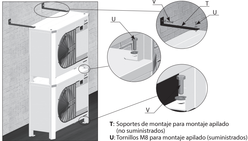
Ilustración 2: Montaje apilado
