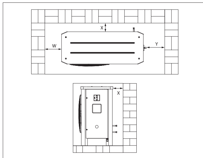
Imagem 1 : Distâncias mínimas de montagem
