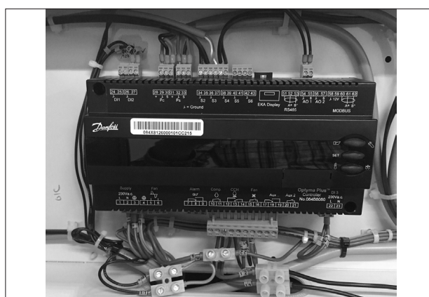
Illustration 5 : Câblage temporaire
