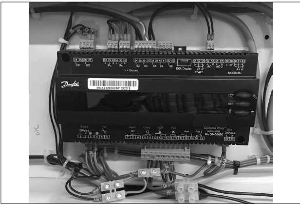
Ilustración 5: Cableado temporal
