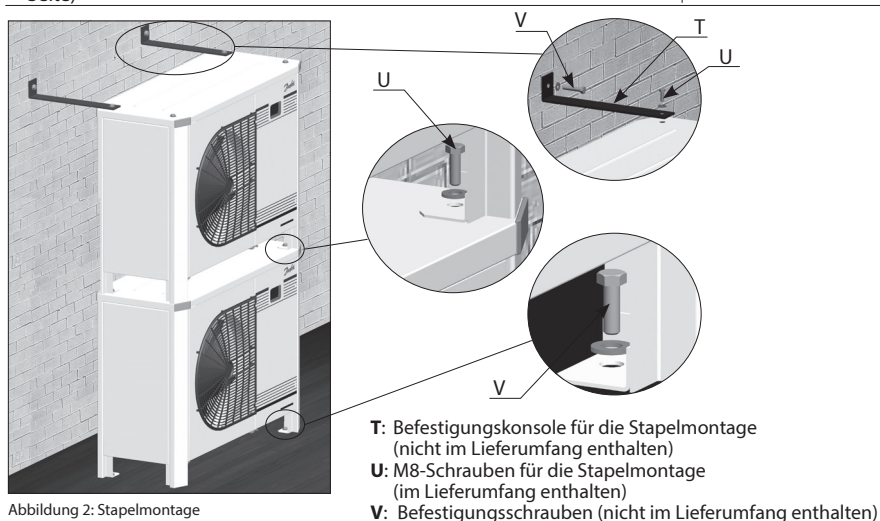
Abbildung 2: Stapelmontage
