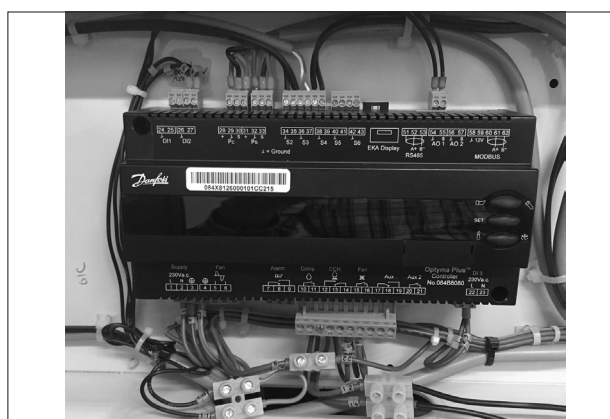
Imagem 5: Cablagem temporária
