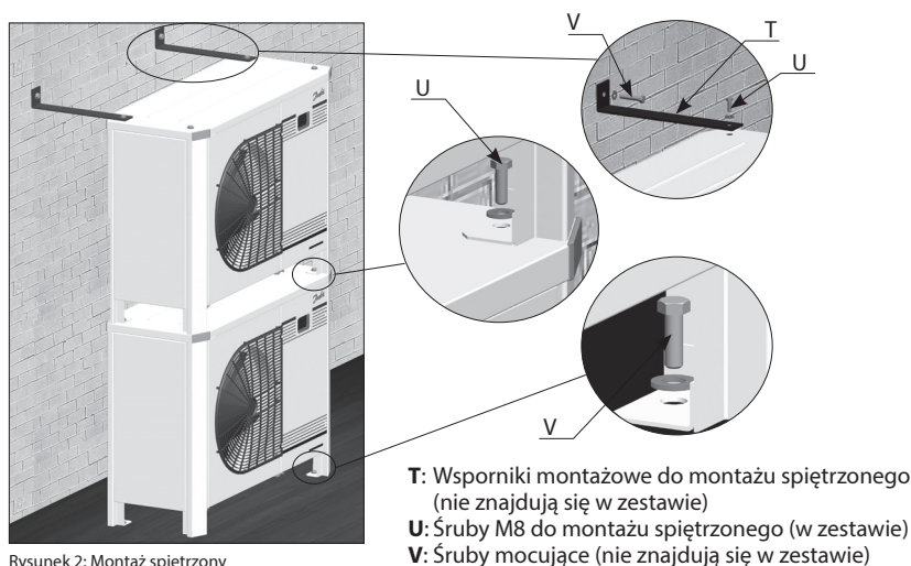
Rysunek 2: Montaż spiętrzony
