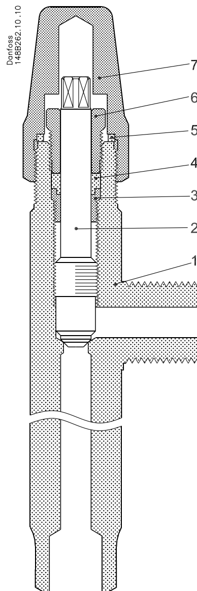
SNV-ST und SNV-SS (Verlängerter Anschluss)
