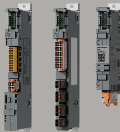
Commande et cartes optionnelles
