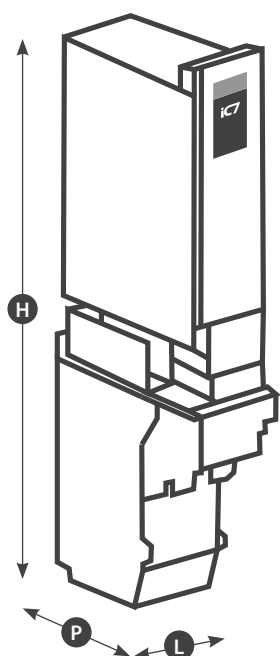
Module avec unité d'intégration standard
