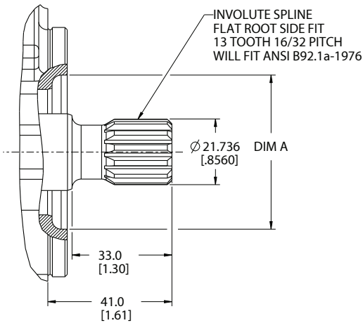
07 - SAE J744-22-4, SAE B, 13T SPLINE
