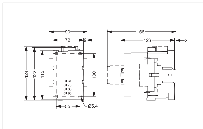
Contactor CI 61, 73, 86, 98
