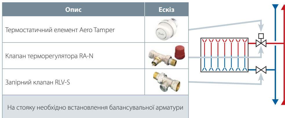
Рис. 8. Приклад комплектації вузла об'язки опалювального приладу в двотрубній системі опалення
