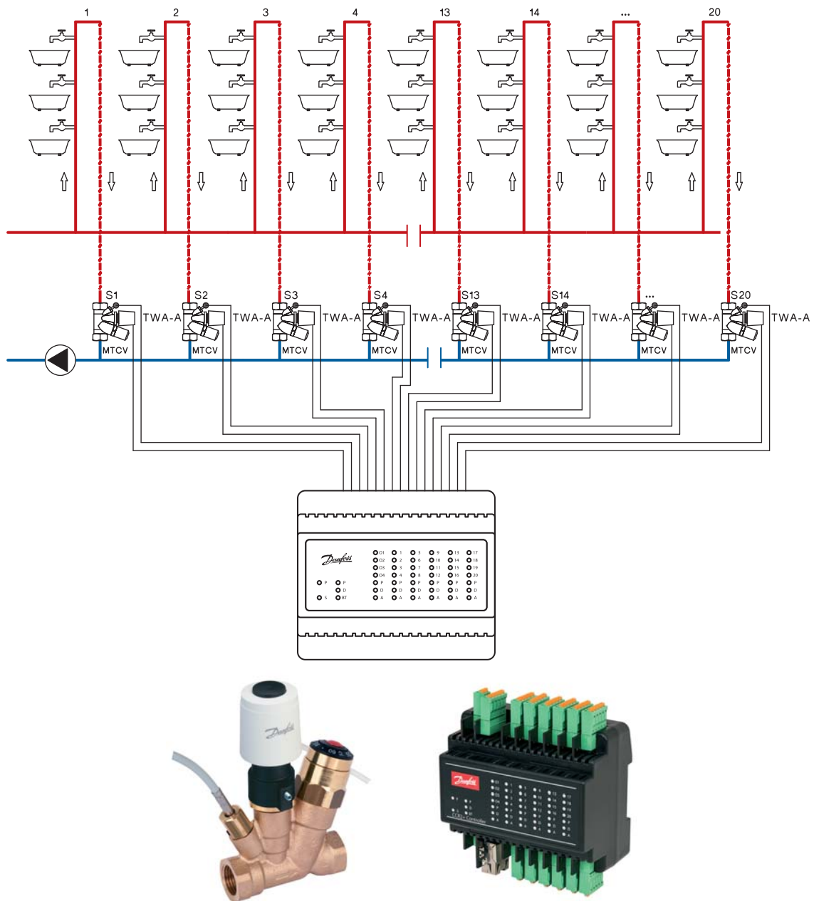
MTCV + TWA-A
