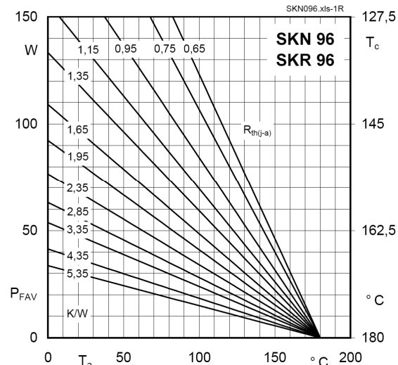
Fig. 1R Power dissipation vs. ambient temperature
