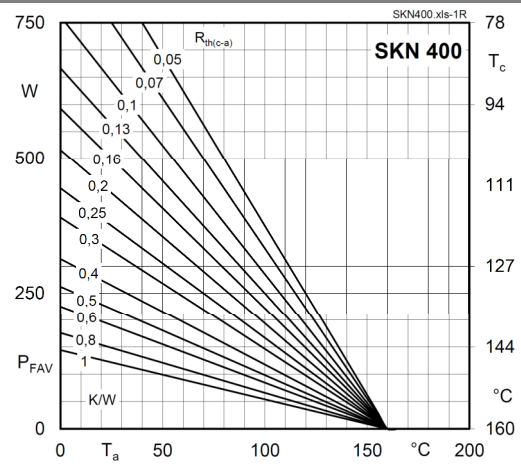
Fig. 1R Power dissipation vs. ambient temperature
