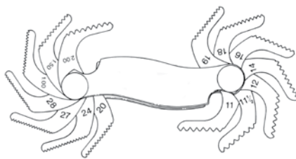
Medidor de paso de rosca
