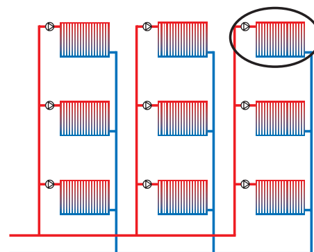
Abb. 6: Messung am hydraulisch letzten bzw. ungünstigsten gelegenen Heizkörperthermostatventil
