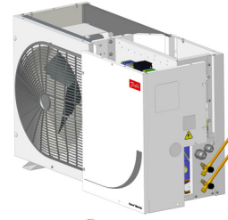
Passo 4: Retire o painel lateral paralelo ao interruptor
