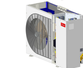
Шаг 4. Снимите боковую панель в направлении, параллельном главному выключателю.
