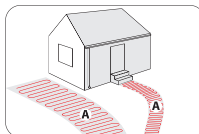
Enkeltzonesystem til færdselsareal (system A)
