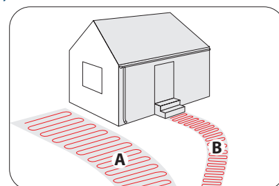
To-zoners system til færdselsareal (system A og B)
