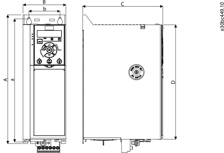
图 1: 机箱规格 J1–J7 的机械尺寸
