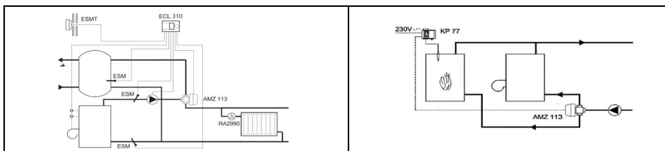
Prednostna priprava sanitarne tople vode - delilni ventil.
