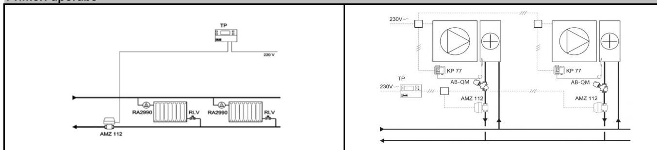
ON-OFF regulacija radiatorskega ali talnega ogrevanja, nočno znižanje.
