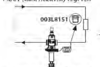
Impulzní trubka připojená na vratné potrubí
