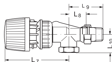
Sensore incorporato RA2000 su valvola RA-FN, a squadra orizzontale
