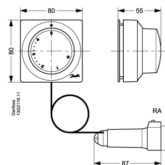
Regolatore remoto della temperatura RA2000
