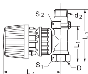
Sensore incorporato RA2000 su valvola RA-FN o RA-G
