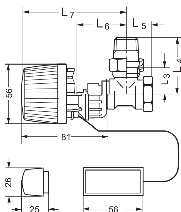
Sensore remoto RA2000 su valvola RA-FN o valvola RA-G
