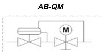
Princíp funkcie
