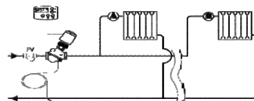
Obj.č. 003L5042 (súčasť balenia) Typická aplikácia
